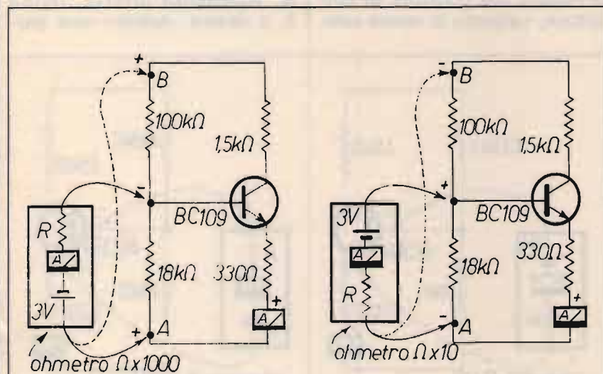
figura 1 Misurazioni ohmetriche sul partitore. A sinistra misuriamo i due resistori del partitore (giunzioni inversamente polarizzate). A destra misuriamo i resistori di emettitore e collettore (giunzioni direttamente polarizzate).
