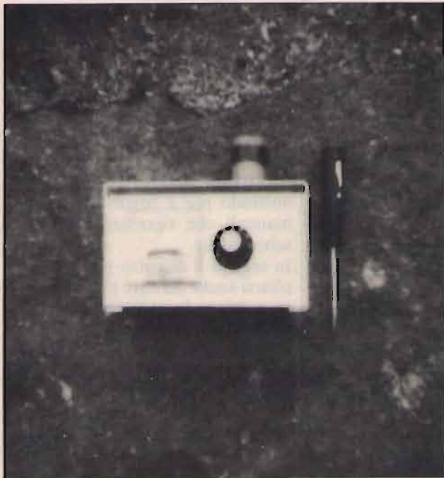
figura 3 Aspetto dell'ondometro a realizzazione ultimata: la bobina-sonda dev'essere applicata sul coperchio del contenitore metallico.
