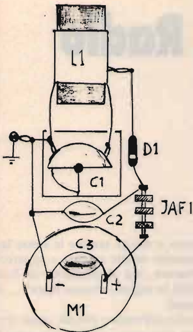
figura 2 Piano di cablaggio dell'ondometro ad assorbimento.
