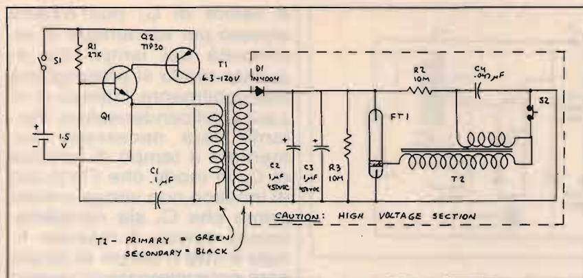
figura 4 Schema di un circuito a lampo singolo.
